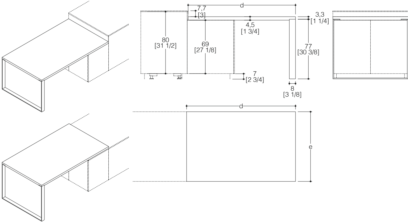
TIPO "C" TYPE "C"
