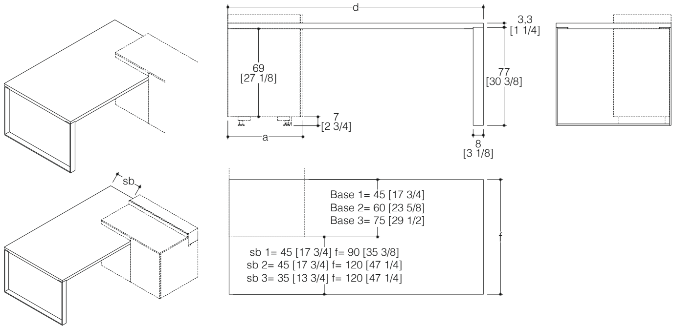
TIPO "D" TYPE "D"
