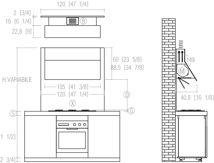
VERSIONE FILTRANTE CON SCHIENALE INOX FILTERING VERSION WITH STAINLESS STEEL WALL PANEL
