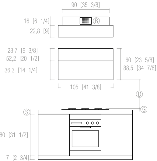
VERSIONE FILTRANTE - FILTERING VERSION
