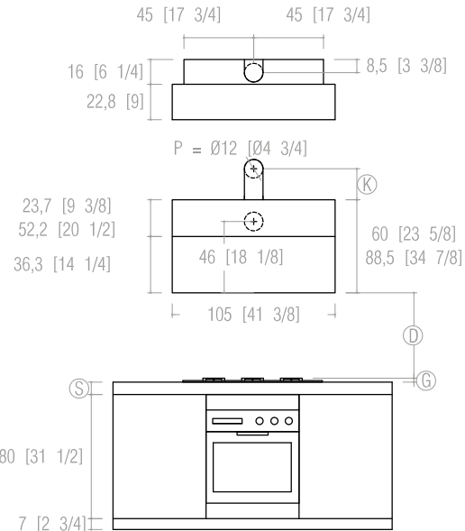
VERSIONE ASPIRANTE - EXTRACTOR VERSION
