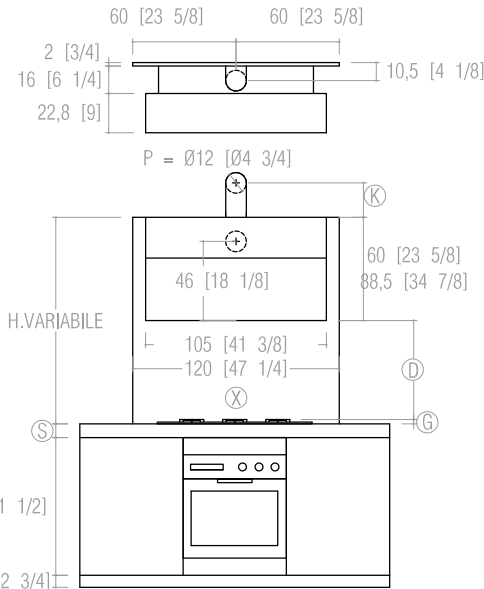
VERSIONE ASPIRANTE CON SCHIENALE INOX EXTRACTOR VERSION WITH STAINLESS STEEL WALL PANEL
